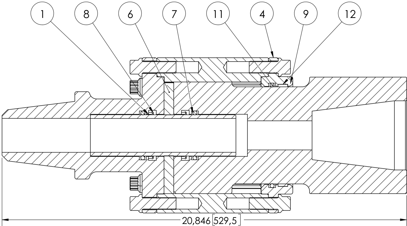
COUPE A-A
